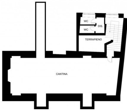
PIANO SOTTOSTRADA SCALA 1:50 FORMATO A2
